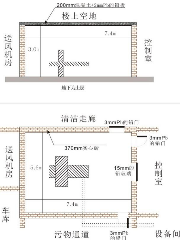
图 10-2 DSA 机房防护设计图
