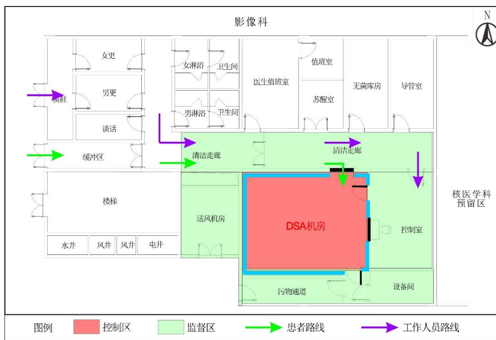
图 10-1 DSA 工作场所分区管理示意图
