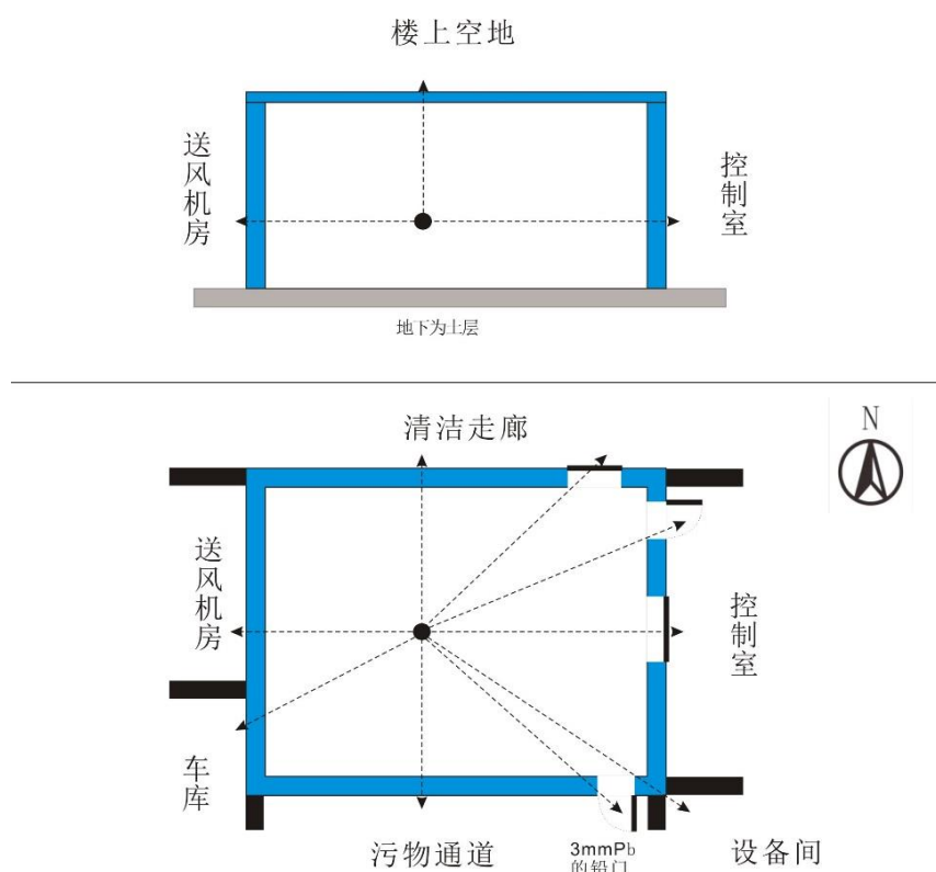
图 11-1 DSA 机房关注点分布简图
