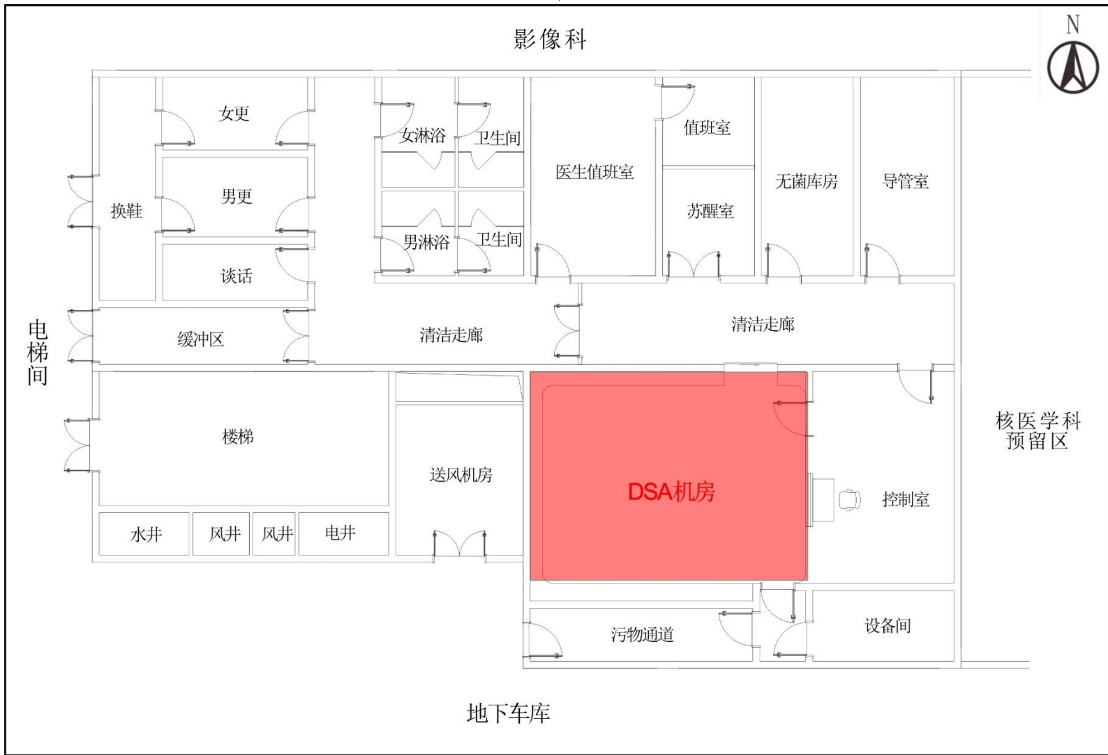
图 1-4 DSA 机房周边关系图
