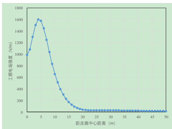
图 6.2-5 1F4-SZ2 型塔弧垂高度 7m 工频电场强度随距离变化趋势
