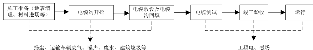
图 4-3 电缆线路施工期、运行期工艺流程及产污环节示意图
