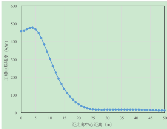
图 6.2-1 1GGF4-SZ2 型直线杆弧垂高度 12m 工频电场强度随距离变化趋势
