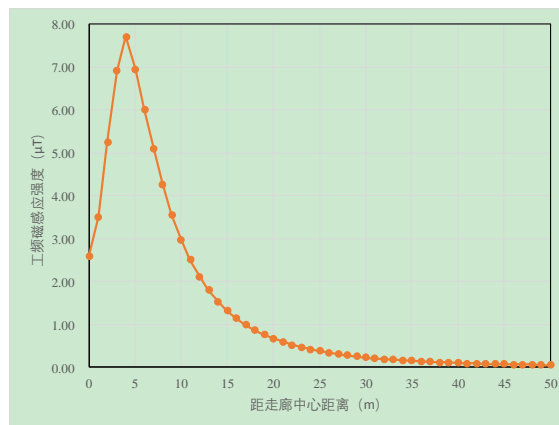
图 6.2-4 1F4-SZ2 型塔弧垂高度 6m 工频磁感应强度随距离变化趋势
