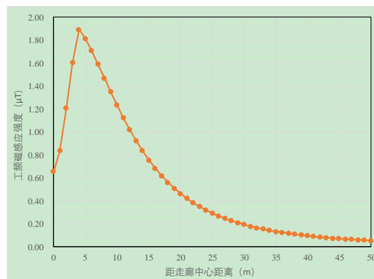
图 6.2-8 1F4-SZ2 型塔弧垂高度 12m 工频磁感应强度随距离变化趋势
